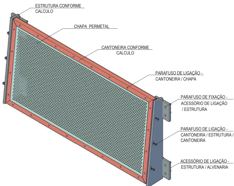
01 DETALHES DE INSTALAÇÃO
