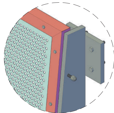
02 DETALHES DE INSTALAÇÃO
