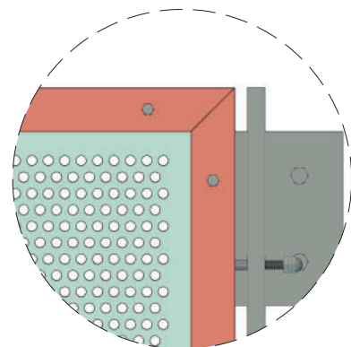
03 DETALHES DE INSTALAÇÃO
